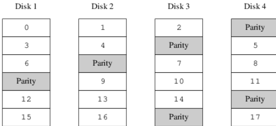
图 105. RAID-5 的组织
